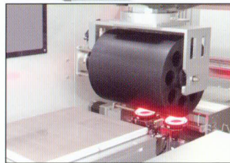
貼付部分拡大写真 Close-up photo of affixer section
